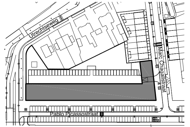
Situatie 1:2000
